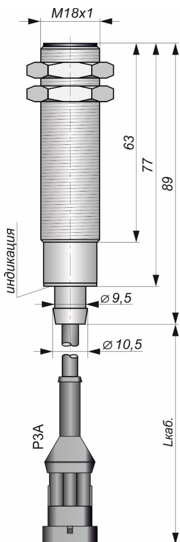
Габаритный чертеж
